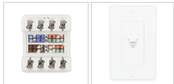
Cat5e 180° Keystone
